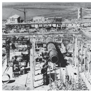
Вид на строительство печного отделения. На заднем плане – цех помола
