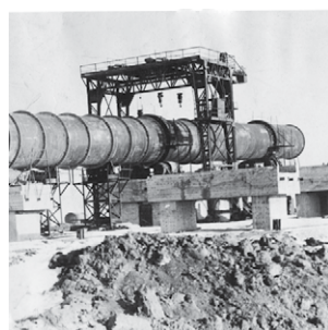
Монтаж корпуса печи, 1961 год
