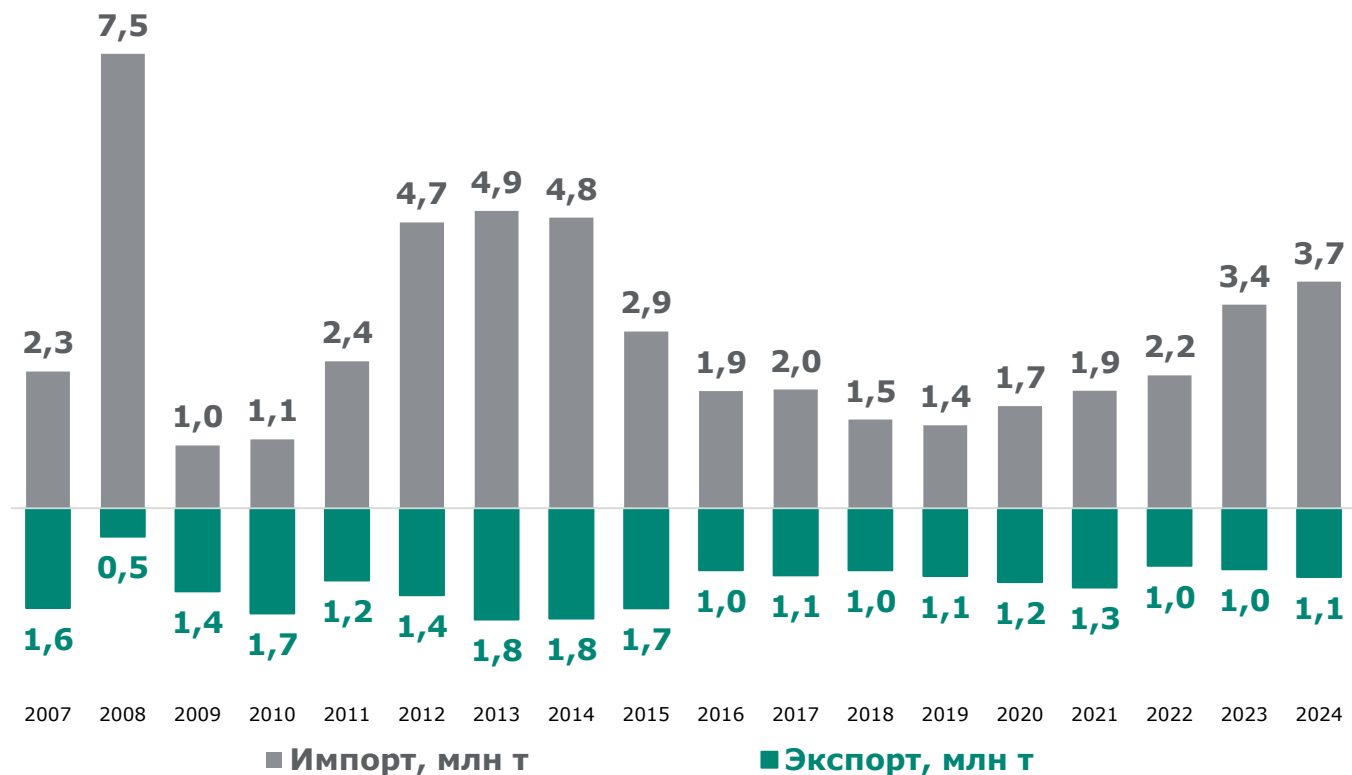
Динамика ввоза и вывоза цемента РФ за январь-декабрь 2024 г., тыс. тонн
